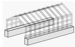
Streifenfundament 2-seitig
