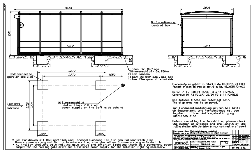
Beispiel eines Fundamentplans
