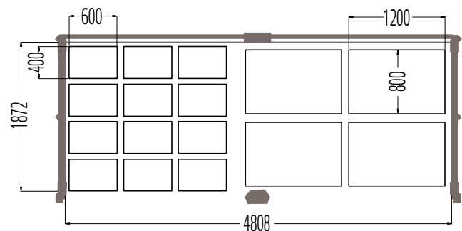
Beispiel-Plan für die praktische Bestückung mit Paletten (Draufsicht)
